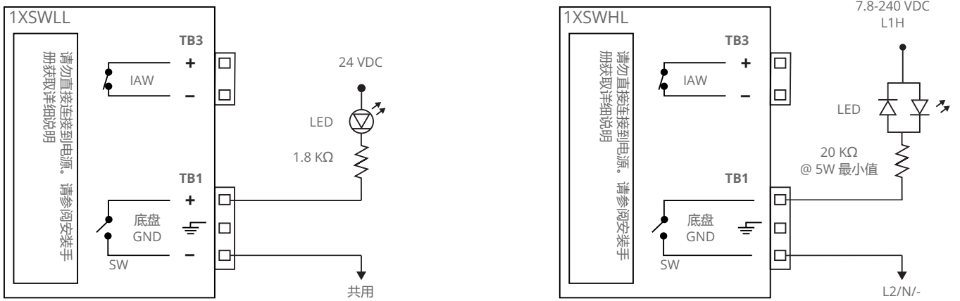
图9 推荐台架测试电路
