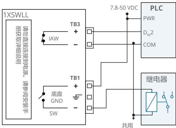
图 7 带 IAW 电路的中间继电器
