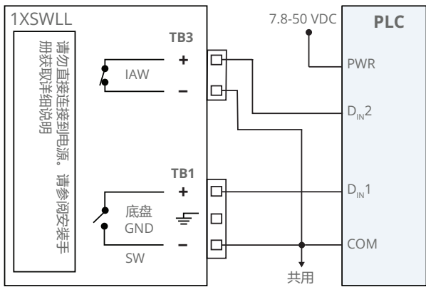
图 5 SW 和 IAW PLC 输入电路
